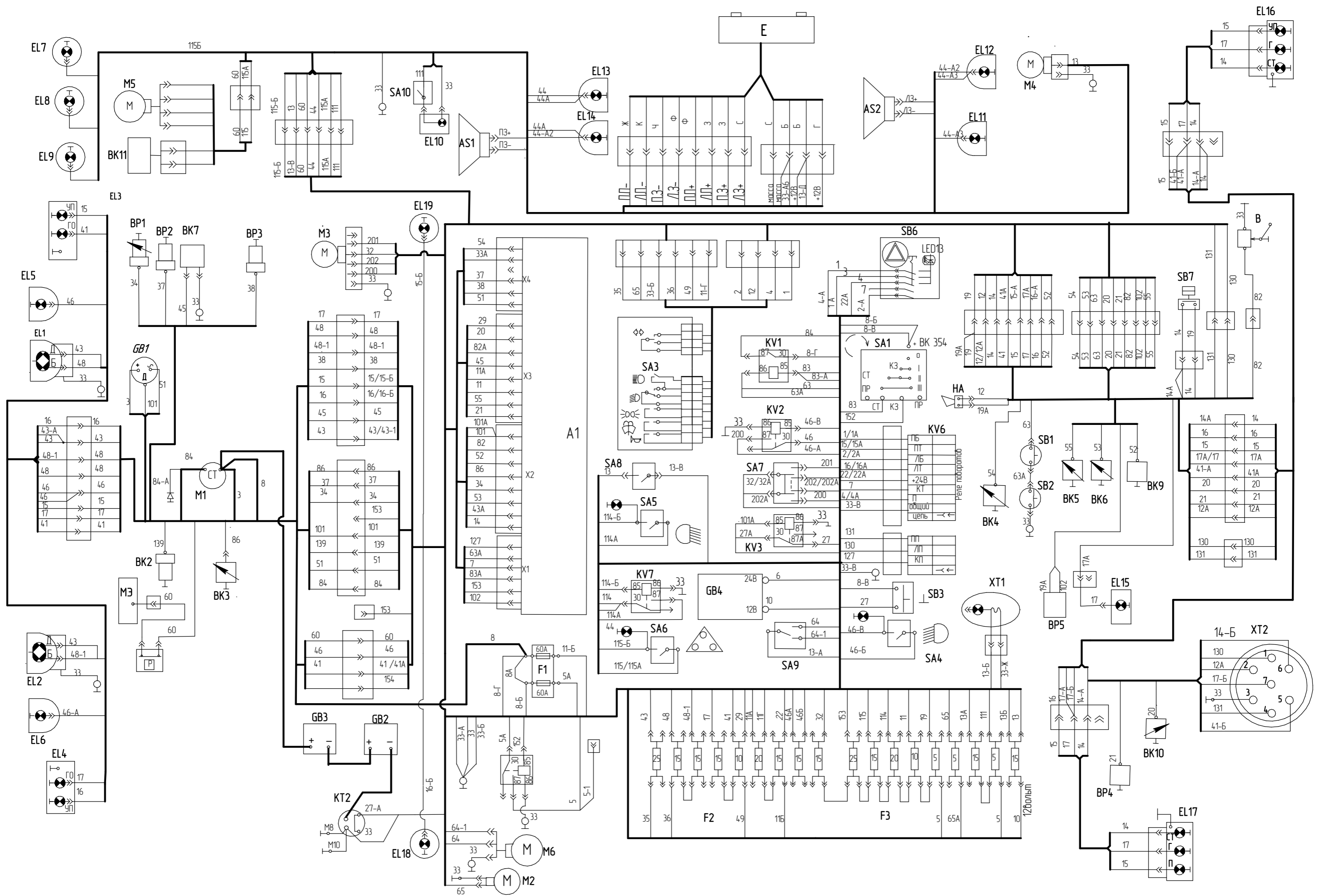
Схема электрическая соединений
